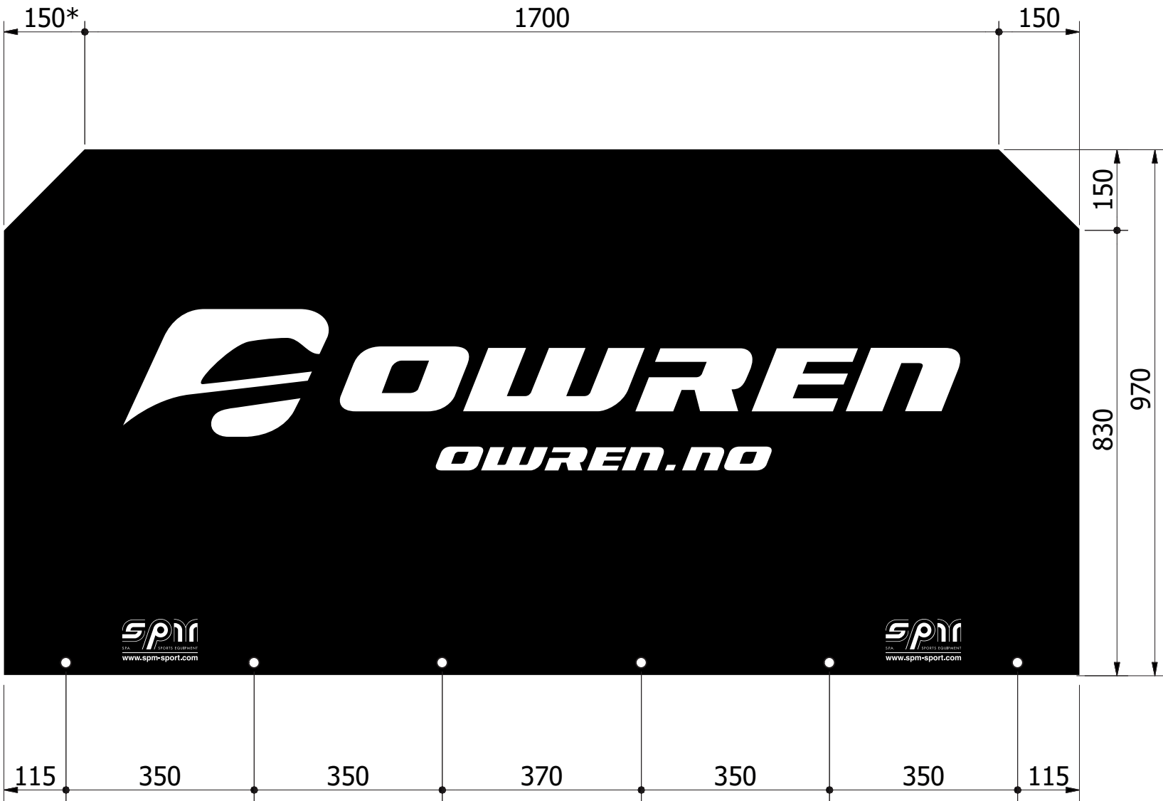
Fronte/Frontscala 1:10
